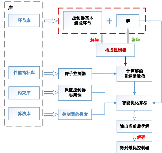
图 8 结构可优化抗扰控制器的设计框架 [107]
