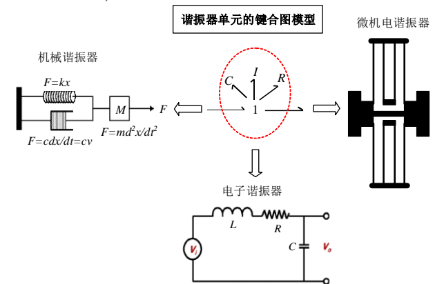
图 5 不同应用领域的谐振器键合图表示
